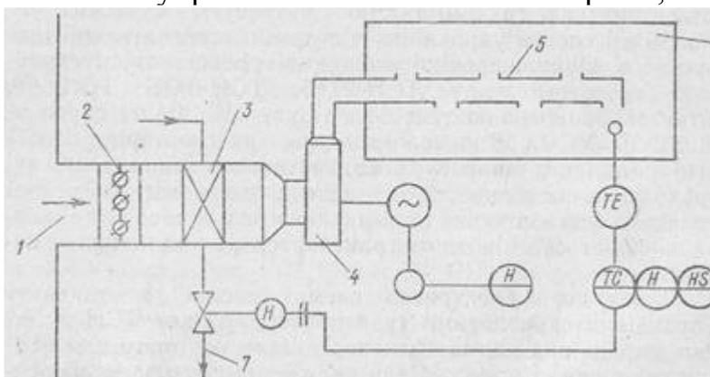
Спрощена електрична принципова схема безперервного регулювання частоти обертання електродвигунів вентиляторів:
