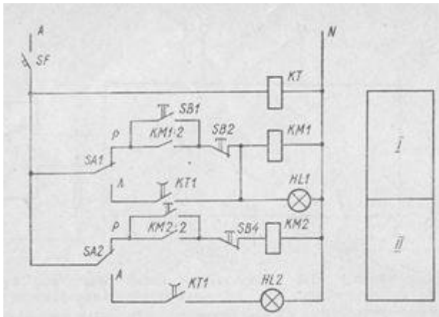
Електрична принципова схема
